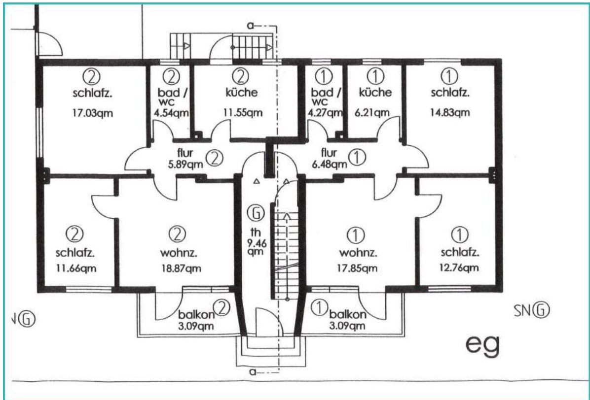
Grundriss Wohnung 1
